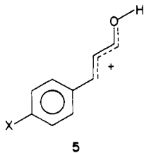
5 a, X=OCH 3 ; b, X=CH 3 ; c, X=H; d, X=F; e, X=CF 3 ; f, X=NO 2
